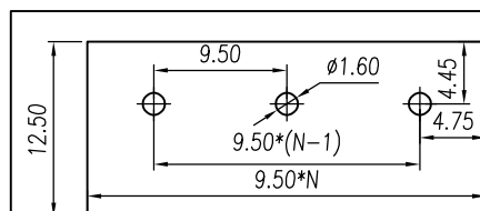
PCB. 钻孔图
